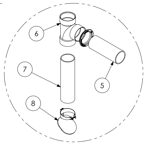
OUTLET ASSEMBLY 2-A
