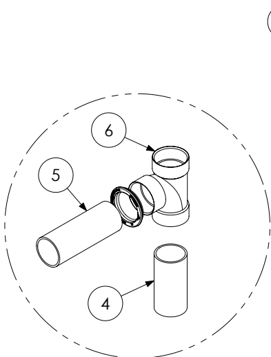
INLET ASSEMBLY 1-A
