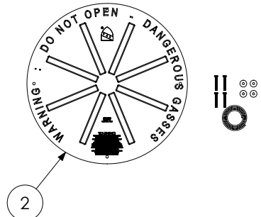
OUTLET ASSEMBLY 2-A
