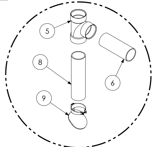
OUTLET ASSEMBLY 2-A
